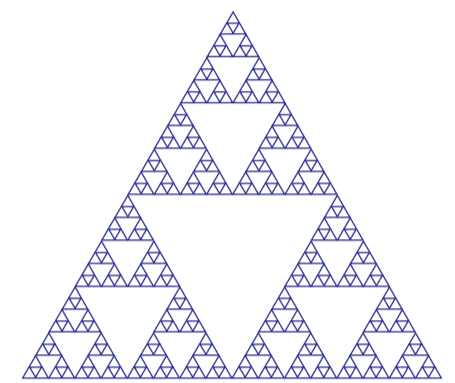
Sierpinski triangle or Sierpinski fractal
